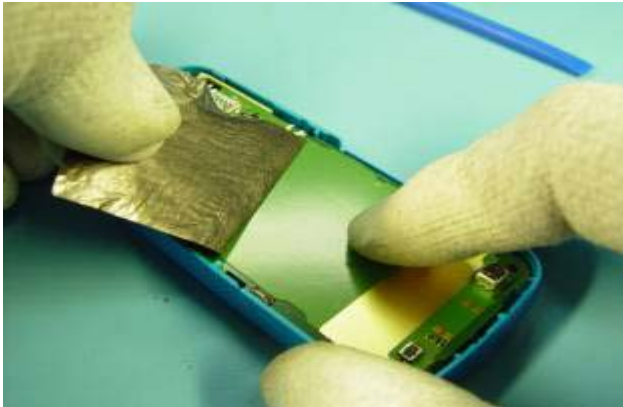
25) Peel up the GT TAPE.
