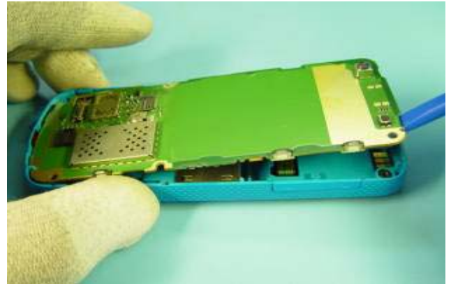
26) Lift out the ENGINE MODULE.
