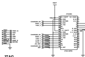
JTAG
