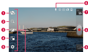
Menu icons
