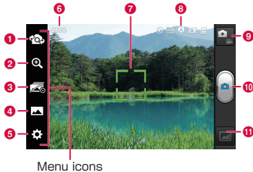
Menu icons
