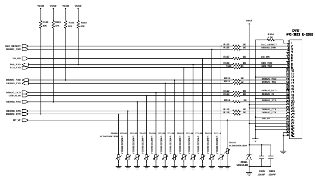
IF CONNECTOR
